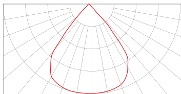
Louver - 80°
